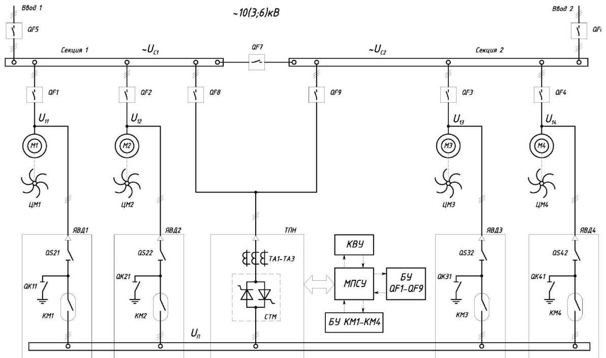
Рис. 1. Электрическая схема автоматизированного плавного пуска группы высоковольтных АЭП центробежных механизмов.
